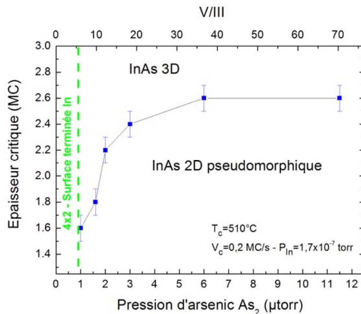
Figure 3.4. Epaisseur critique H_{3D} en fonction de la pression d'arsenic ( \text{As}_2 ) pendant la croissance, pour T_c=510^\circ\text{C} et V_c=0,2 MC/s.
