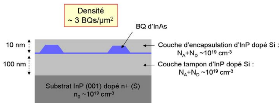
Figure 4.12. Schéma de la structure à boîte dopée aux électrons préparée par SS-MBE
