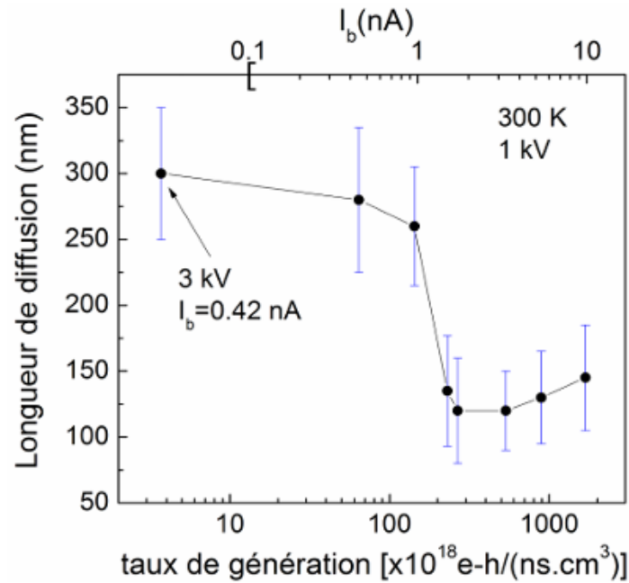
Figure 4.9. Longueur de diffusion en fonction du taux de génération et du courant sonde à 1 kV et 300 K. Une mesure a été faite à 3 kV et 0,42 nA. Les barres d'erreurs correspondent à la déviation standard à la moyenne.
