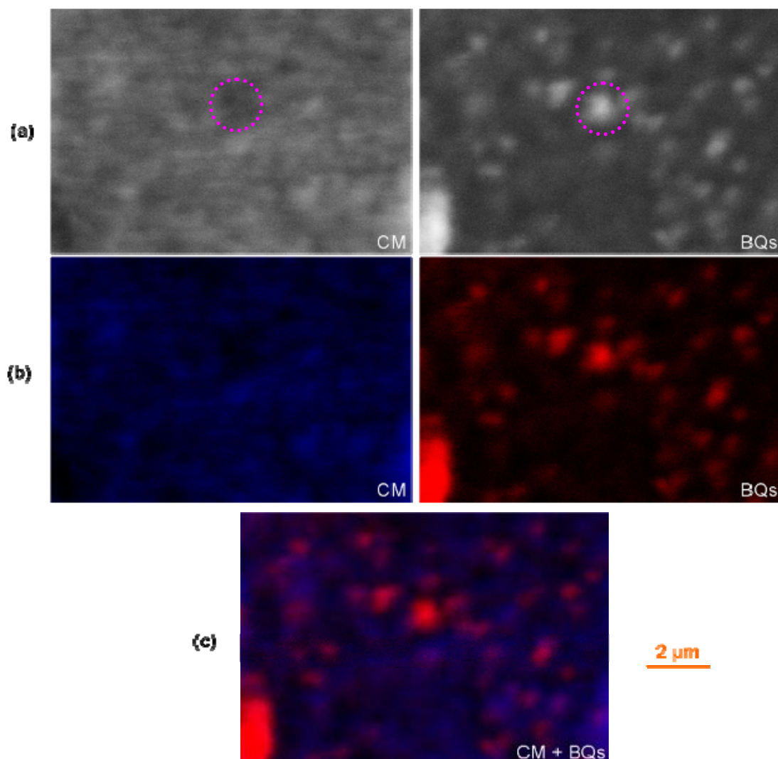
Figure 4.6. (a) Images CL de la couche de mouillage (CM) à 980 nm (fentes 20/40 μm), et de toutes les boîtes détectables en mode panchromatique + filtre, obtenues à 5K. (b) Ces mêmes images colorisées en bleu et rouge respectivement avec un contraste rehaussé afin de mieux distinguer les zones lumineuses. (c) Superposition des images de la CM et des boîtes montrant des anti-corrélations spatiales.
