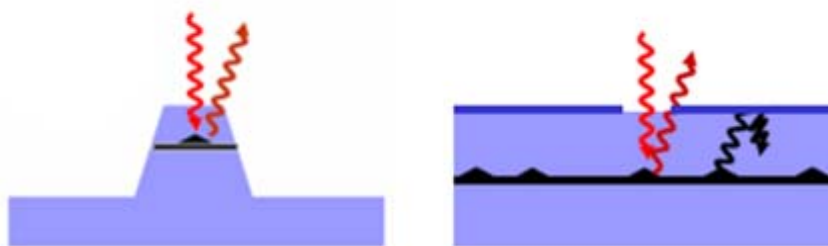
Figure 2.13. Deux techniques d'isolation spatiale de boîtes (a) par la gravure d'un mesa et (b) par une ouverture submicronique dans un masque métallique. L'excitation du laser est en rouge et la luminescence des boîtes isolées spatialement est représentée en magenta. L'émission des boîtes en dehors de l'ouverture (en noire) est bloquée par le masque.
