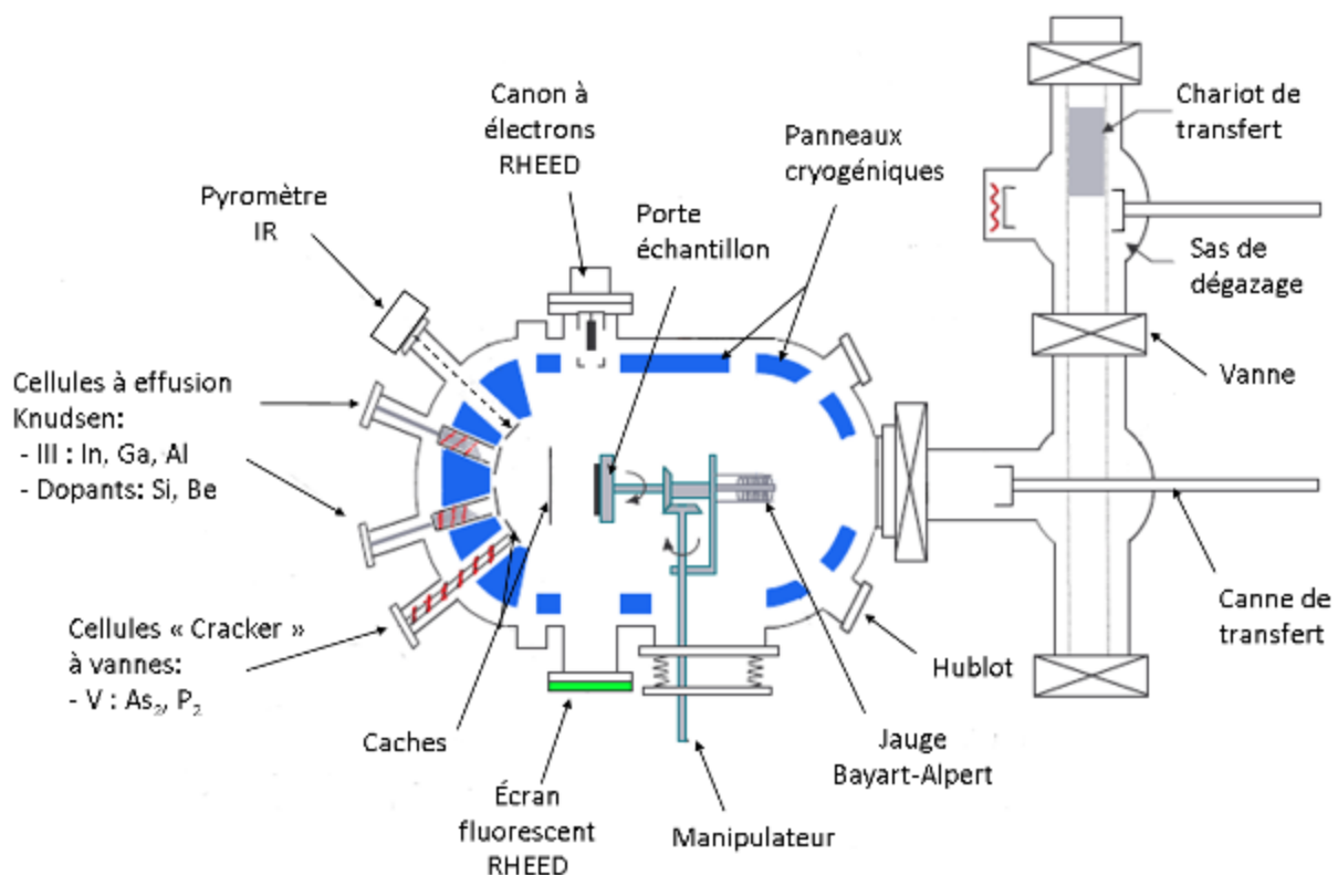
Figure 2.1. Diagramme schématisique du réacteur d'épitaxie Riber 2300 en coupe transversal. Le système des pompes à vide est situé en dessous.
