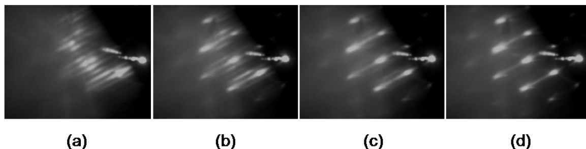
Figure 3.22. Echantillon A : Diagrammes RHEED suivant [1\bar{1}0] (a) des bâtonnets ( E_{\text{InAs}} = 1,6 \text{ MC} ) après 10 s de recuit à 520^\circ\text{C} puis (b-d) pendant la descente en température sous une forte pression d' \text{As}_2 : (b) T = 460^\circ\text{C} , (c) T = 430^\circ\text{C} , (d) T = 400^\circ\text{C} .
