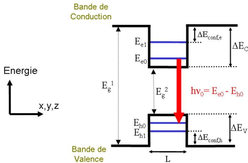
Figure 1.2. Diagramme de bande schématisant d'une boîte quantique semi-conductrice de bande interdite directe E_g^2 enterrée dans une matrice de plus grande bande interdite E_g^1 . Les valeurs indiquées sont pour : la largeur du puits ( L ), la séparation entre la bande de valence et de conduction des deux matériaux ( \Delta E_C et \Delta E_V ), les niveaux d'énergie pour les électrons et les trous ( E_e et E_h ) dans la boîte quantique, l'énergie de confinement pour les électrons et les trous ( \Delta E_{\text{conf},e} et \Delta E_{\text{conf},h} ), la fréquence de transition optique du niveau fondamental ( \nu_0 ).
