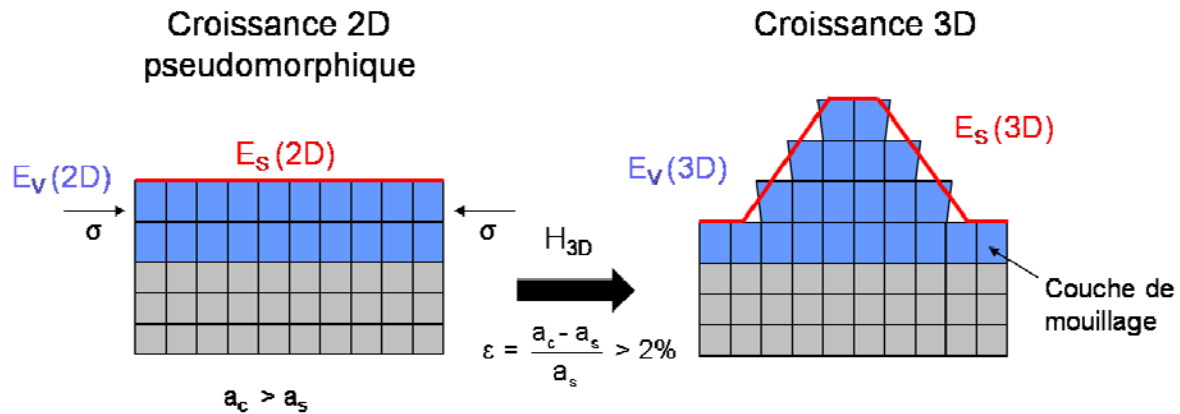
Figure 1.6. Principe de croissance d'îlots quantiques 3D par le mode de croissance Stranski-Krastanov.
