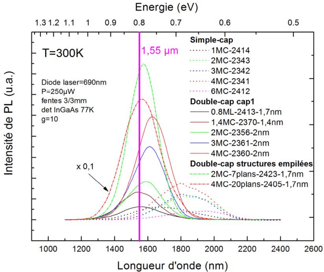
Figure 3.40. Spectres de PL à 300 K des boîtes formées selon la « voie B » avec une encapsulation d'InP soit « simple-cap », soit « double-cap » pour des structures à 1 plan de boîtes et des structures empilées à 7 et 20 plans de boîtes. La densité de boîtes est modifiée avec l'épaisseur d'InAs déposée entre 0,8 et 6 MC. La longueur d'onde d'émission visée est 1,55 μm et l'épaisseur du premier cap est d'environ 1,7 nm.
