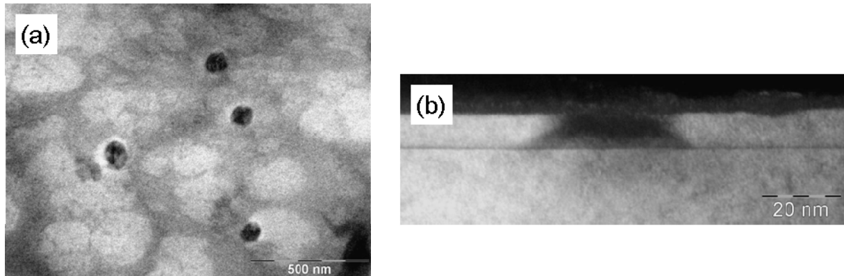
Figure 3.21. Images TEM d'îlots formés par refroidissement sous arsenic à 400°C : (a) vue plane (îlots non capés) et (b) en coupe transverse suivant (îlots capés par 10 nm d'InP). L'épaisseur d'InAs déposé était de 1,4 MC.
