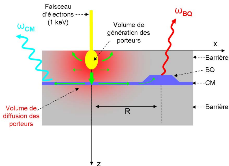
Figure 4.7. Représentation schématique de la mesure de longueur de diffusion des porteurs par une boîte unique.
