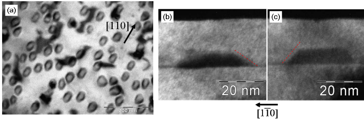
Figure 3.15. Images TEM (a) en vue plane et (b-c) en coupe transverse selon [1\bar{1}0] d'îlots fabriqués selon la voie C et capées par de l'InP à environ 520°C. L'épaisseur d'InAs déposée est égale à 2 MC.
