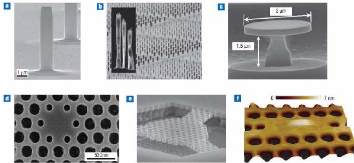
Figure 1.12. Images MEB de cavités semi-conductrices. (a)-(b) micropiliers, (c) microdisque, (d)–(f) cristaux photoniques planaires. D'après [Shields 07].
