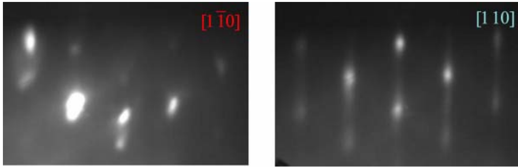
Figure 4.15. Images RHEED suivant [1\bar{1}0] et [110] de la surface d'InAs après 4 min de recuit sous As à 510°C. Les taches lumineuses indiquent clairement la formation de boîtes.
