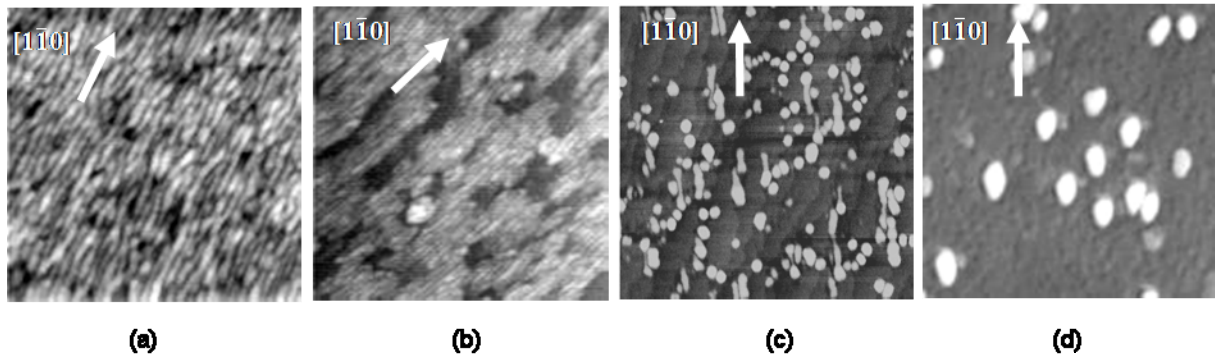
Figure 3.19. Images AFM ( 1 \mu\text{m} \times 1 \mu\text{m} ) d'îlots montrant l'évolution morphologique des bâtonnets crûs à 520°C (a) au cours de la descente en température ( \sim -30^\circ\text{C}/\text{min} ) sous flux d'arsenic. La commutation As/P pendant la descente en température permet de geler la morphologie de surface à environ (b) 460°C, (c) 430°C, (d) 400°C.
