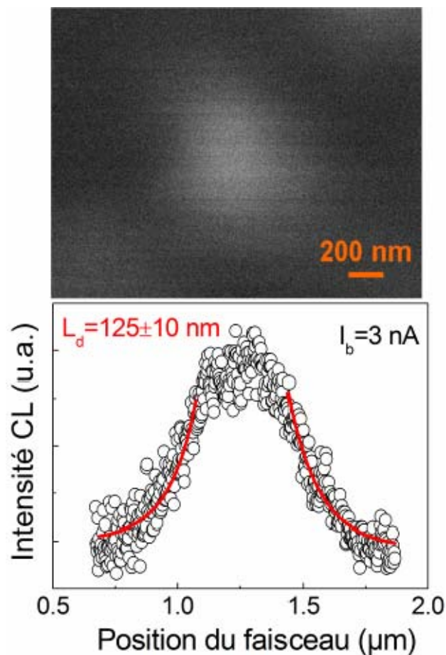
Figure 4.8. (a) Image CL d'une boîte unique en mode panchromatique à 1 keV, 3 nA, 300K. La zone balayée fait environ 1,6 \times 1,2 \mu\text{m}^2 . (b) Profil d'intensité suivant [100] lissé par la fonction en 1/\text{csch}(R/L_d) qui permet d'extraire L_d .
